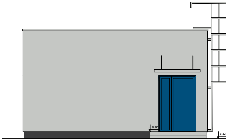
Elewacja frontowa
